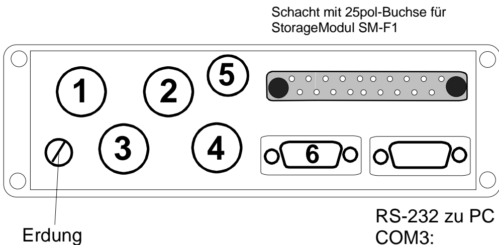
Bild 16: Anschluss-Buchsen im Überblick (mit internem GSM-Modem)
