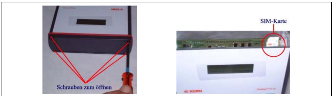
Bild 25: Deckel öffnen und SIM- Karte einführen
