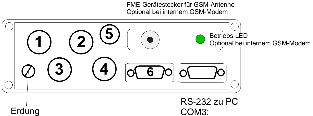
Bild 16: Anschluss-Buchsen im Überblick (mit internem GSM-Modem)
